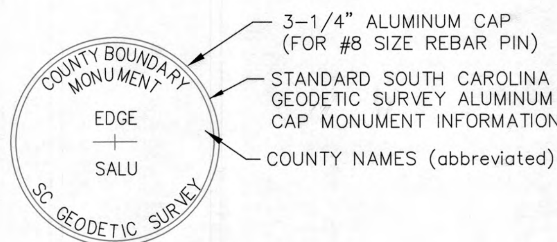
SURVEY MARKER CAP DETAIL (N.T.S.)
